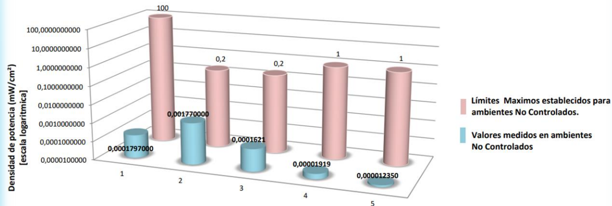
Límites establecidos de densidad de potencia y rangos de valores medidos
